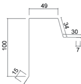
1. Päätysta, pystysaumakatteet, L = 3000 mm
