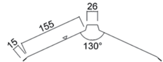
4. Harjalista sileä, L = 30000 mm
