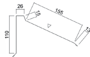
9. Pulpettikaton ylärästästalista, L = 3000 mm
